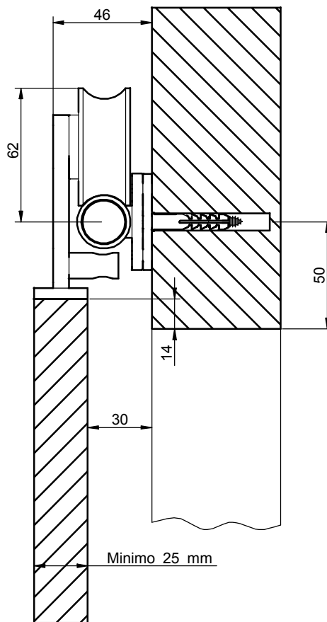
FIJACION TRASERA PARED / Back fixing wall / Fixation l'arriere sur mur
